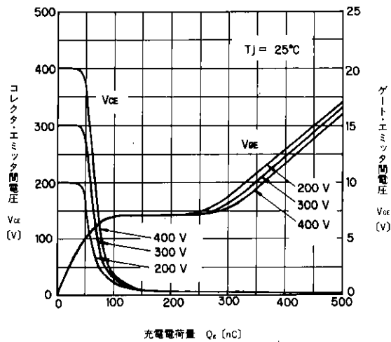
ダイナミック入力特性
