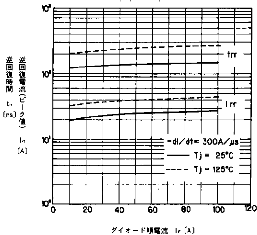
t_{rr} , I_{rr} - I_f 特性
