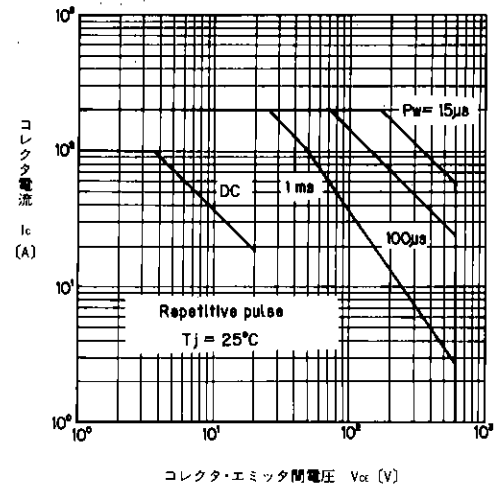
安全動作領域(繰り返し)
