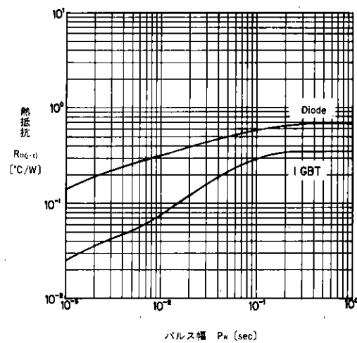
過渡熱抵抗
