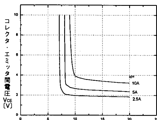
コレクタ・エミッタ間電圧-ゲート・エミッタ間電圧特性 ( T_j=125^\circ\text{C} ) <ブレーキ部> Collector-Emitter voltage vs. Gate-Emitter voltage <BRAKE>
