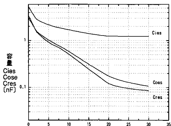
容量-コレクタ・エミッタ間電圧特性 ( T_j=25^\circ\text{C} ) <INV部> Capacitance vs. Collector-Emitter voltage <INV>
