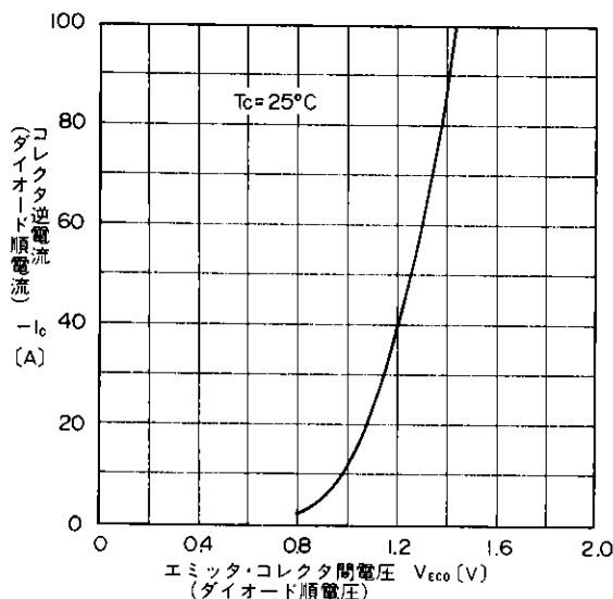
エミッタ・コレクタ間電圧 V_{ce} (V) (ダイオード順電圧) 高速フリーホイーリングダイオード順電圧 Forward Voltage of Free Wheeling Diode
