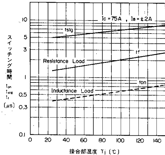
スイッチング時間 接合部温度 T_j ( ^\circ\text{C} ) Switching Time
