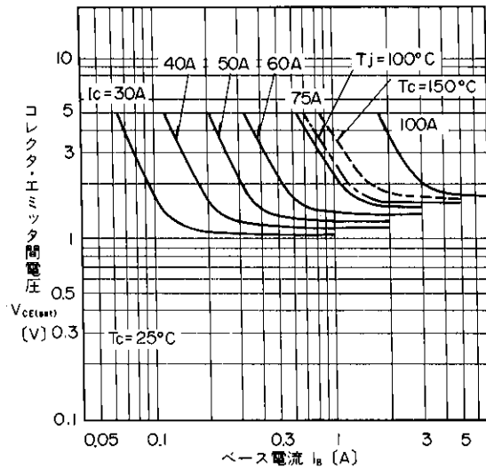
出力特性
