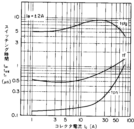
スイッチング時間 コレクタ電流 I_c (A) Switching Time
