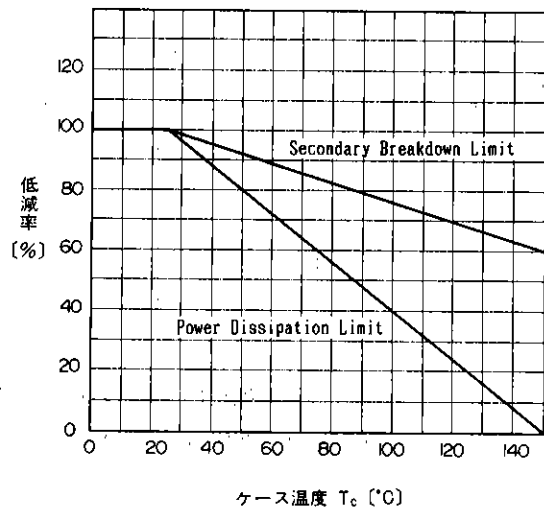
ケース温度 T_c ( ^\circ\text{C} ) ASO 低減特性 ASO Derating
