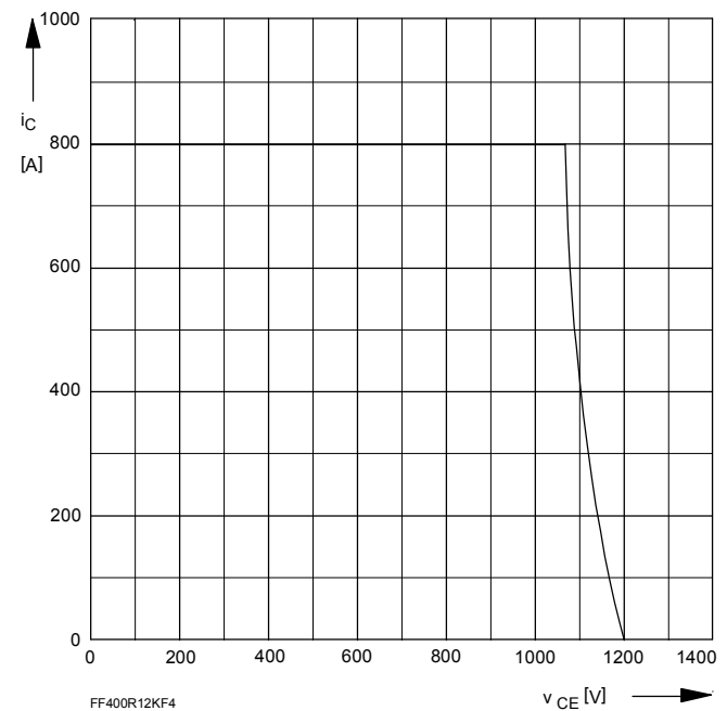
Bild/Fig. 4 Rückwärts-Arbeitsbereich Reverse biased safe operating area t_{vj} = 125\text{ °C} , v_{LF} = v_{LR} = 15V , R_G = 3,6\text{ W}
