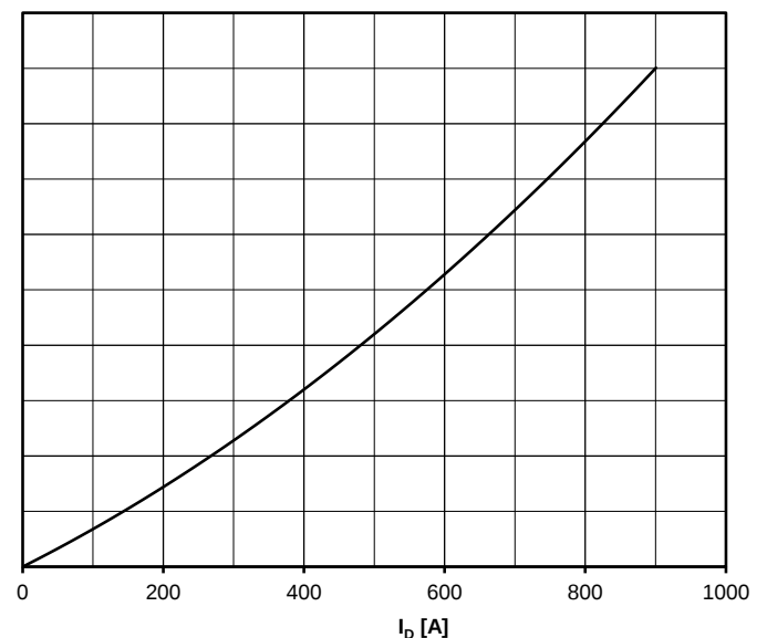
Höchstzulässiger Ausgangsstrom / Maximum rated output current I_D
